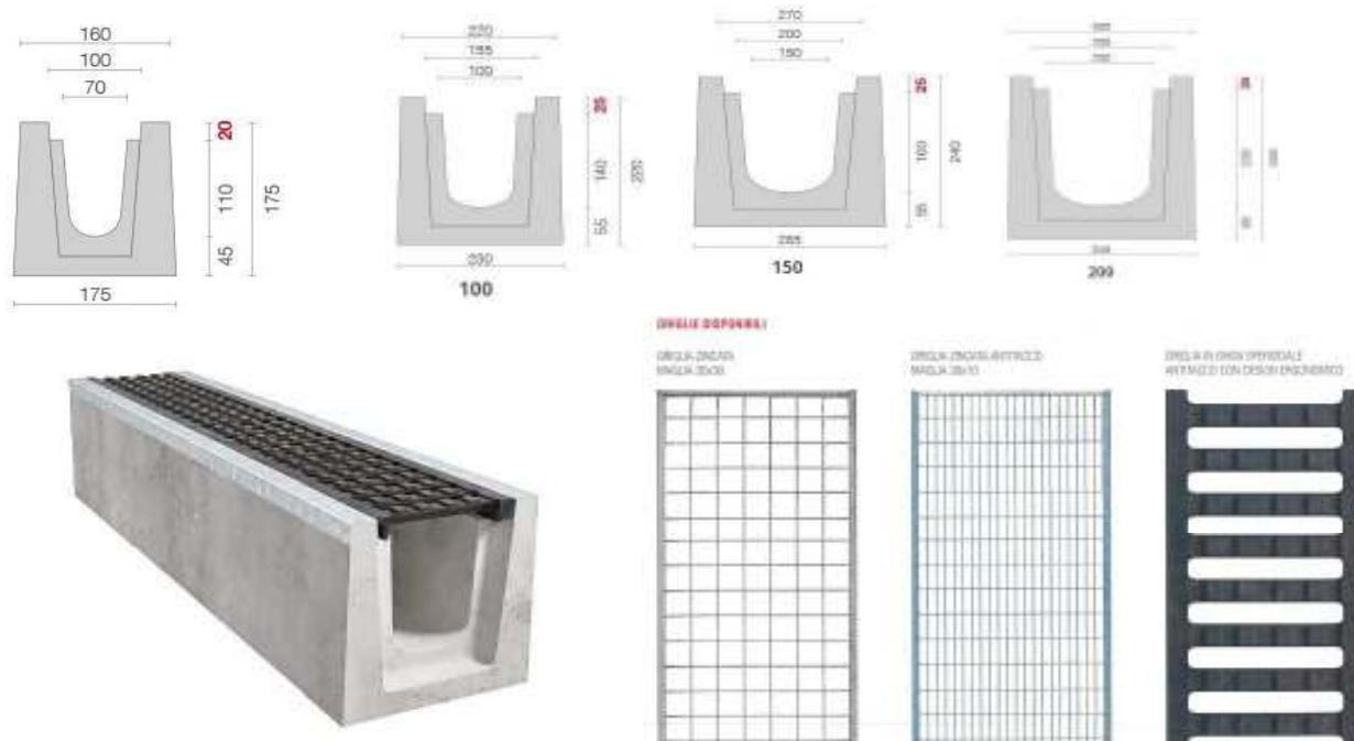
Canala classica con bordo in cls o bordo zincato, con griglia ad incastro.
